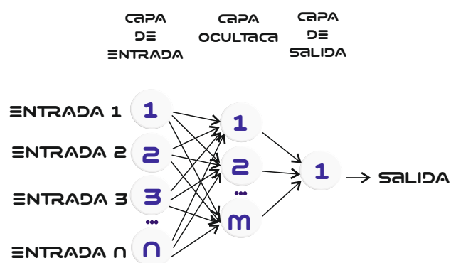
Figura: Red neuronal artificial con una capa de entrada de "n" neuronas, una capa oculta de "m" neuronas y una capa de salida con solo una neurona, de Gengiskanhg. Wikipedia en español. CC BY-SA 3.0.
